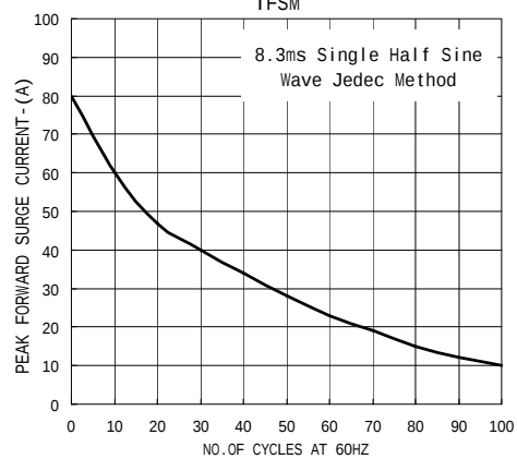
IFSM
