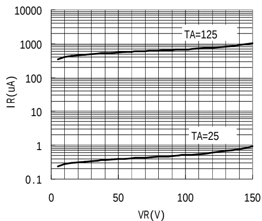
IR - VR
