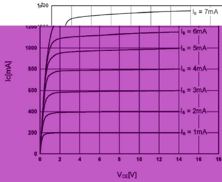
I_C - V_{CE}
