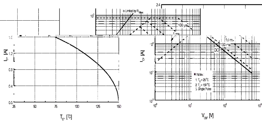
I_D - T_C
