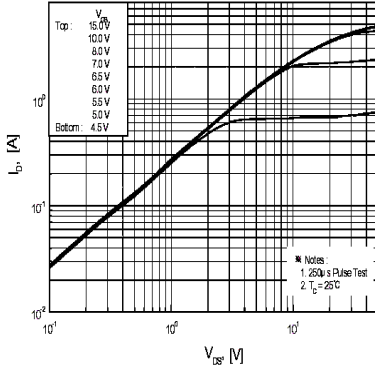
I_D - V_{DS}
