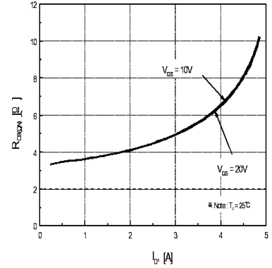
R_{DS(on)} - I_D
