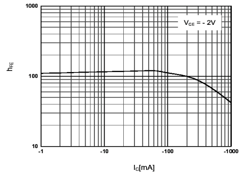
h_{FE} - I_C
