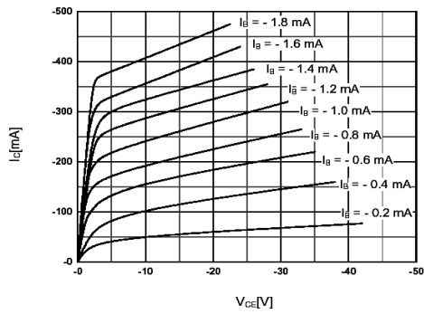
I_C - V_{CE}
